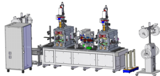
线性工位生产系统方案
