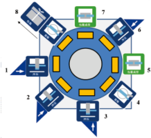
环形工位生产系统方案
